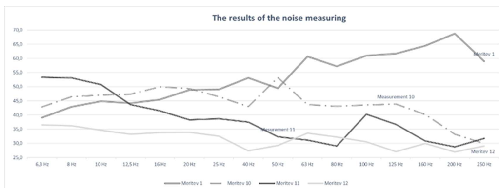
Slika 4. 9: Meritev 1, 10, 11 in 12. NFH izražen kot L_{z\max} na posameznih tercah v intervalu 6,3 – 250 Hz.
