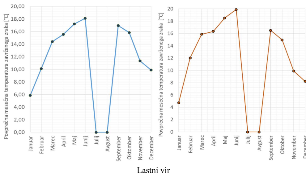
Slika 2.8: Izračunane mesečne povprečne temperaturne zavrženega zraka (a) z računalniškim programom (b) v realnem okolju
