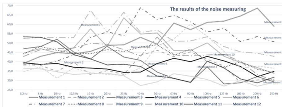
Slika 4. 3: NFH izražen kot L_{Z\max} na posameznih tercah v intervalu 6,3 – 250 Hz, vse merilne pozicije 1.–12.
