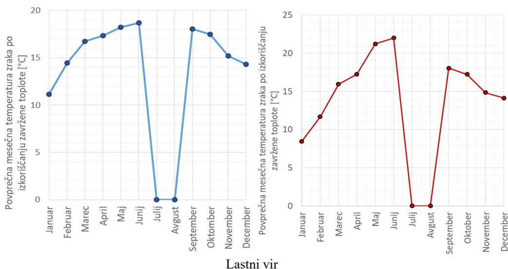
Slika 2.7: Izračunane mesečne povprečne temperature zraka po izkoriščanju zavržene toplote (a) z računalniškim programom (b) v realnem okolju
