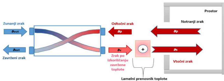
Slika 2.3: Prikaz mehanskega prezračevalnega sistema s prenosnikom toplote za izkoriščanje zavržene toplote
