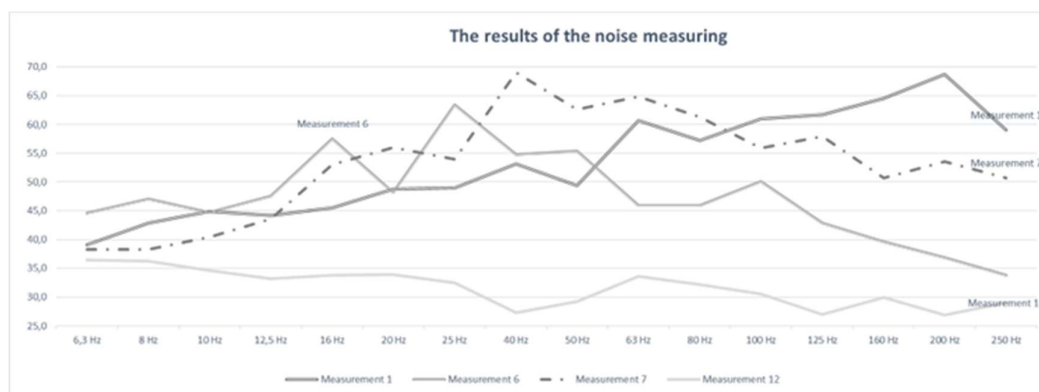
Slika 4. 7: Meritev 1, 6, 7 in 12. NFH izražen kot L_{Z_{max}} na posameznih tercah v intervalu 6,3 – 250 Hz.
