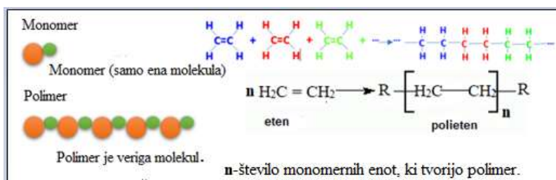
Slika 7.1: Polimerizacija monomera v polimer
