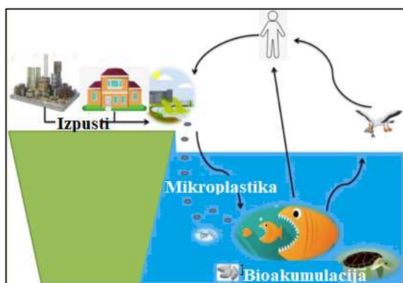
Slika 7.7: Življenjski cikel mikroplastike v okolju
