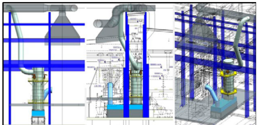
Slika 4: Prikaz umestitve vodno hlajenega hladilnega stolpa (Vir: Erb, Feucht, 2024)
